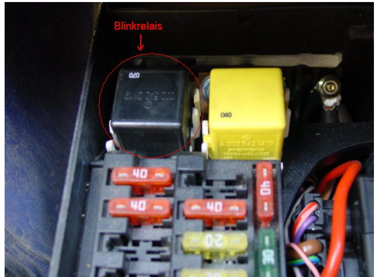
Relaisanordnung beim FaceLift
